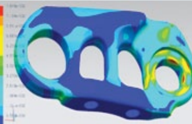
Acople de las orugas
